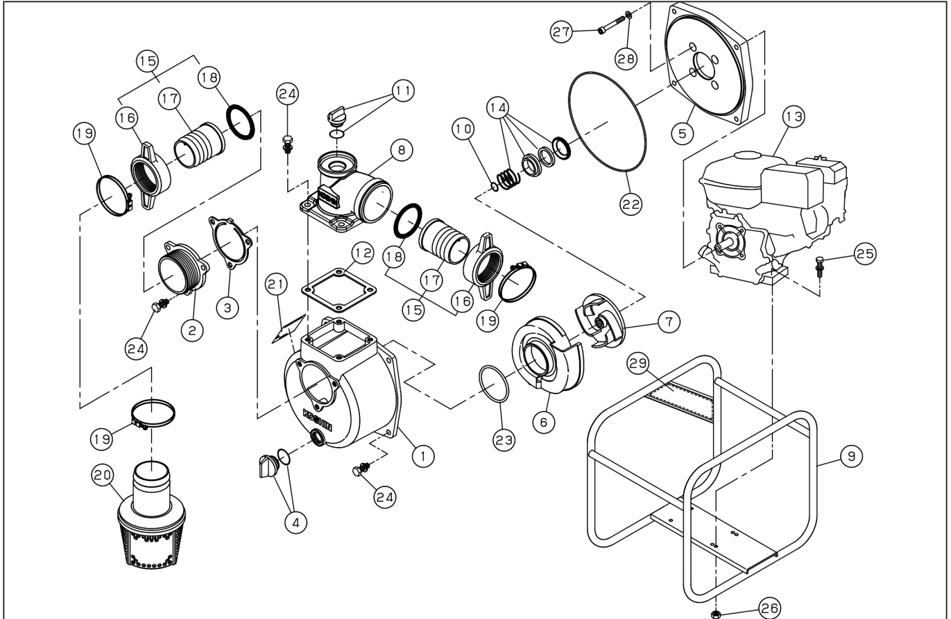
DWG No.011978026 MODEL : SEH-80X FORM : SEH-80X-BBU-6
