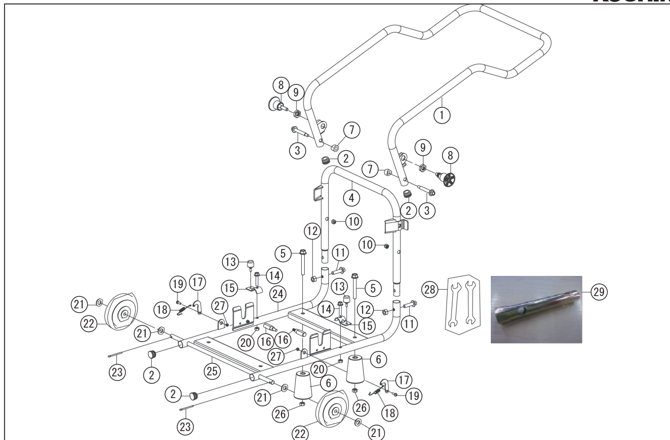
型式名 GVC-1-AAA-0 (065857401) GV-16I 用キャリアセット
