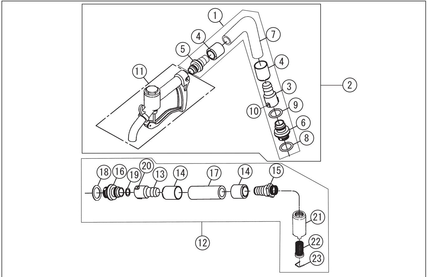
型式名 GM-25 E 型ホースセット (015853203)
