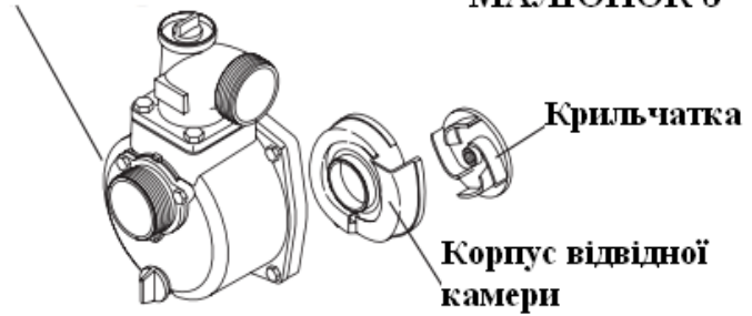
Корпус помпи
