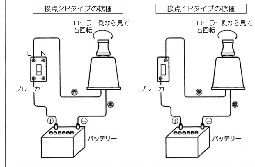
図2・配線例
