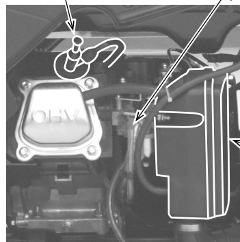
点火プラグキャップ
