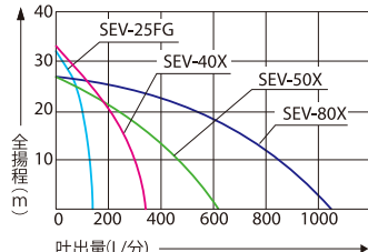
■性能曲線
