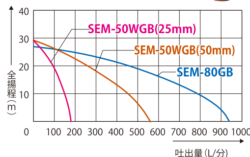
■性能曲線
