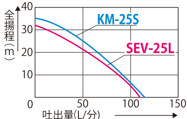
■性能曲線
