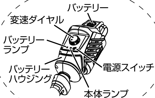
バッテリー取付け部 SBC-1825Lの場合
