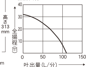
■性能曲線
