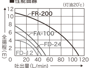
■性能曲線
