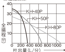
■性能曲線
