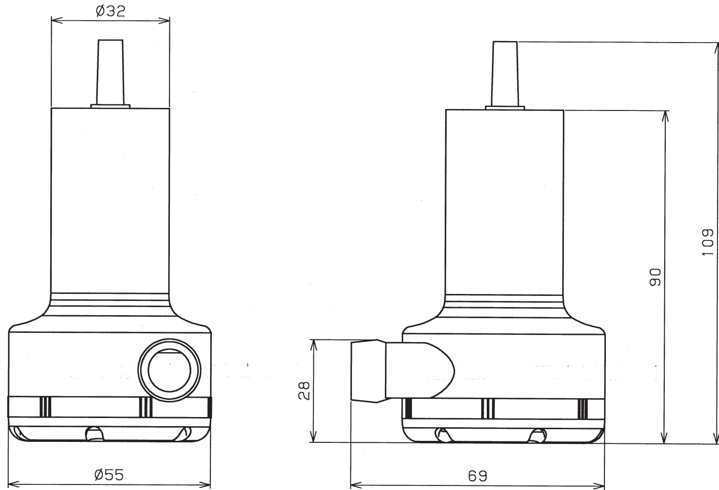
KP-104 ポンプ
