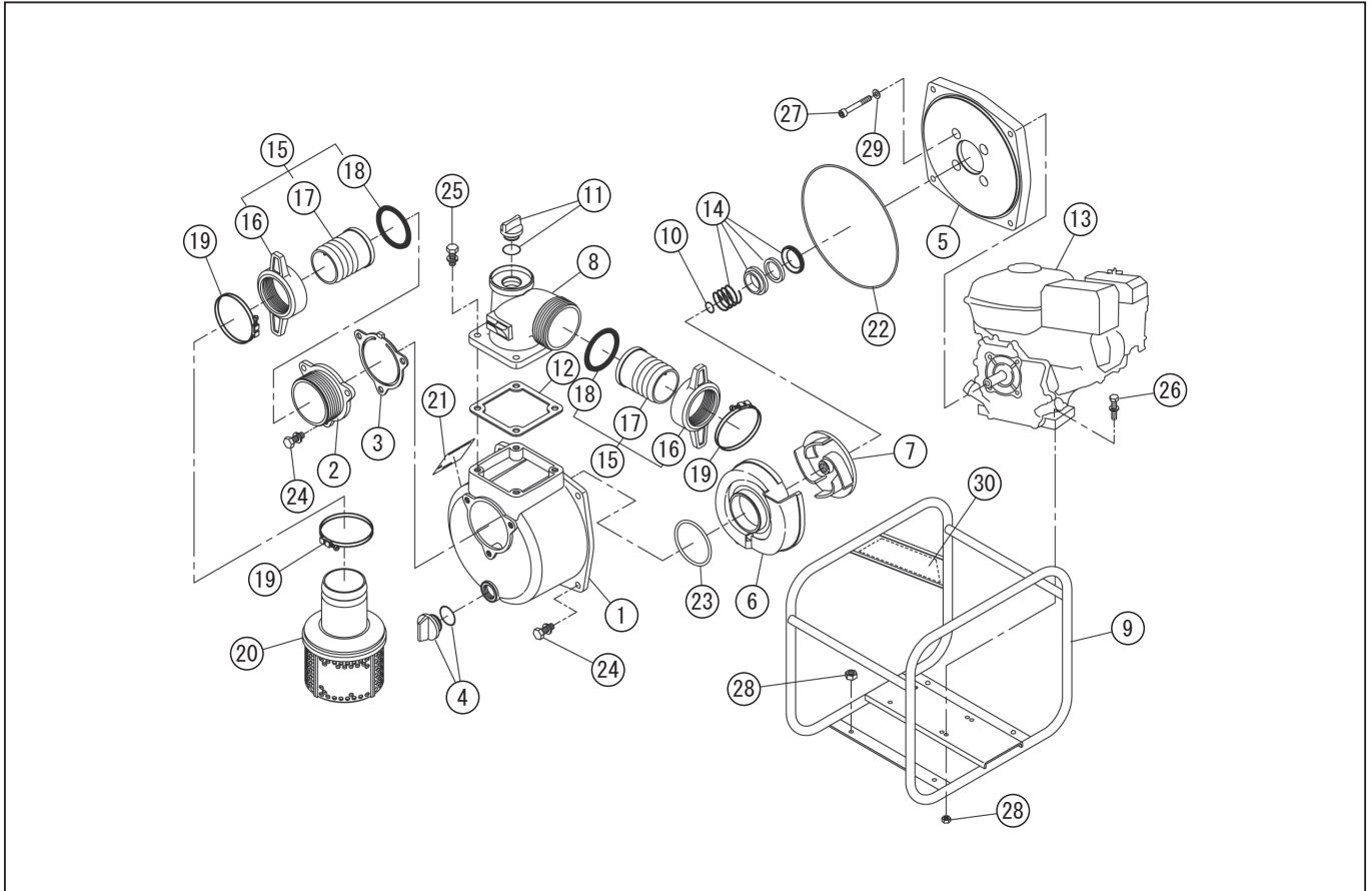
DWG No.012924404 MODEL : SEH-80X FORM : SEH-80X-BFJ-1
