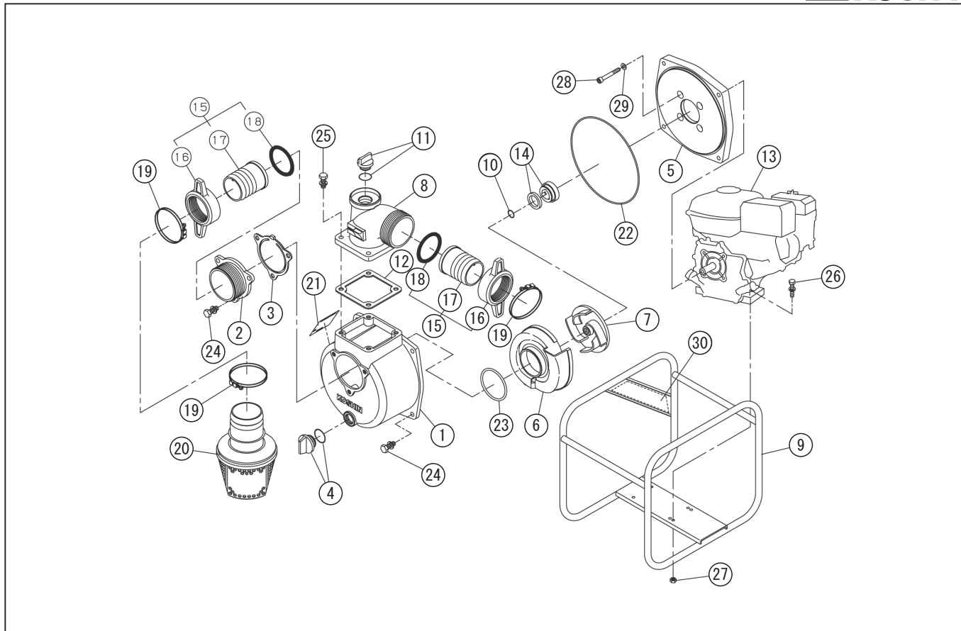
DWG No.012935201 MODELE: STV-80E FORM: STV-80E-BAA-0
