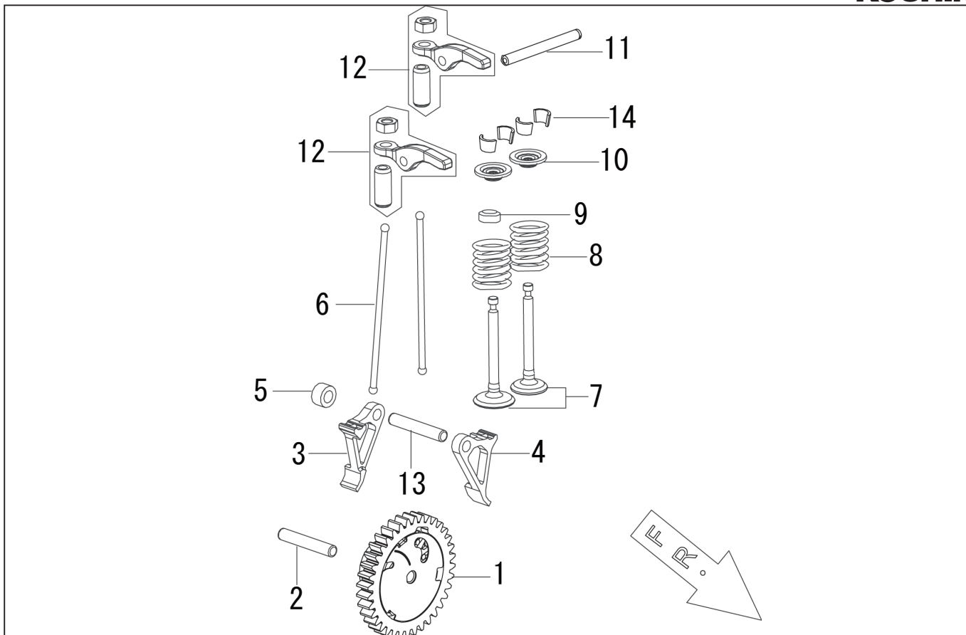
型式名 GV-16SE-AAA-0 (065864601) バルブ、カムシャフト
