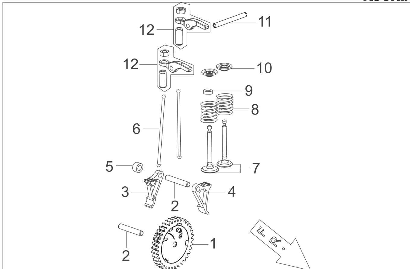
型式名 GV-9IG-AAA-0 (065864401) バルブ、カムシャフト
