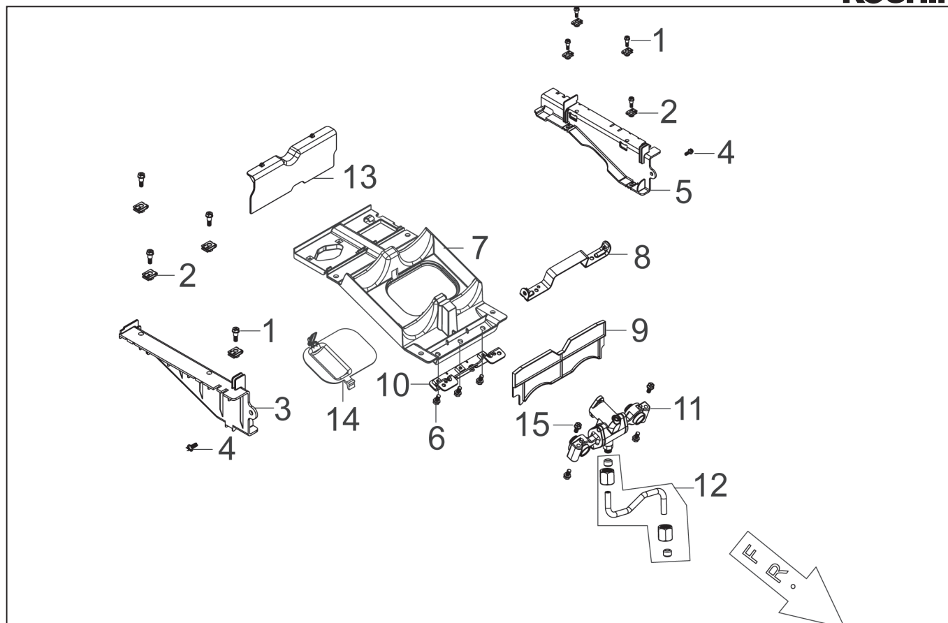
型式名 GV-9IG-AAA-0 (065864401) ボンベカバー内部
